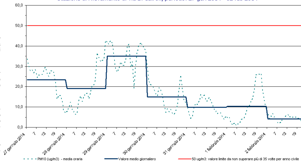
PM10 Stazione di rilevamento di via B. Cairoli, periodo: 27 gen 2014 - 02 feb 2014
