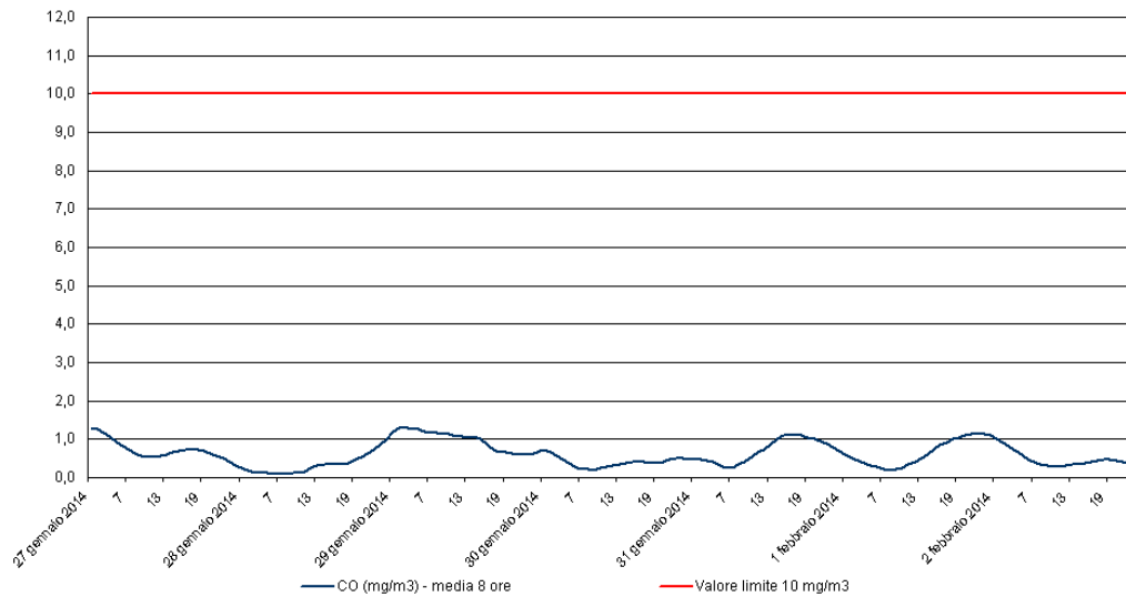
Monossido di Carbonio - CO Stazione di rilevamento di Sambruson, periodo: 27 gen 2014 - 02 feb 2014
