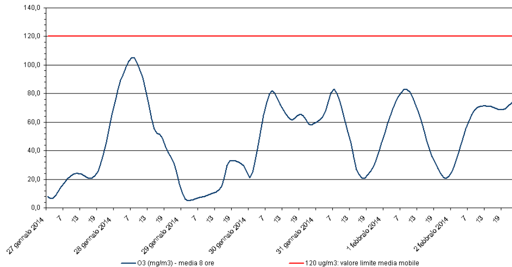
Ozono - O 3 Stazione di rilevamento di Sambruson, periodo: 27 gen 2014 - 02 feb 2014
