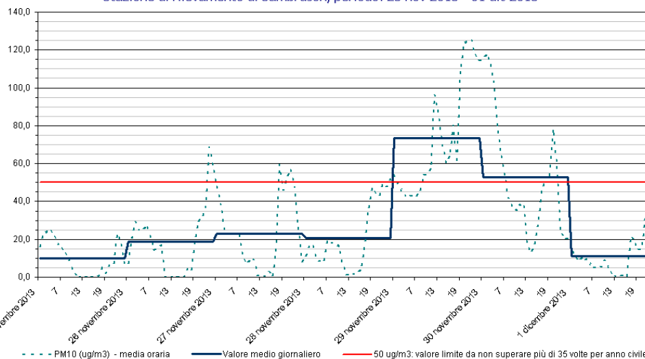
PM10 Stazione di rilevamento di Sambruson, periodo: 25 nov 2013 - 01 dic 2013
