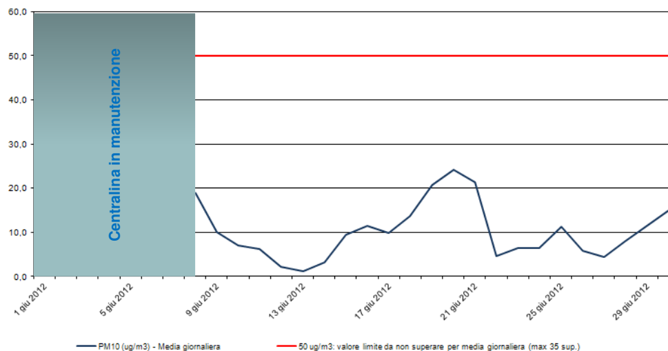
PM 10 Stazione di rilevamento ETL01322 in loc. Palù, periodo: 01 giu 2012 - 30 giu 2012
