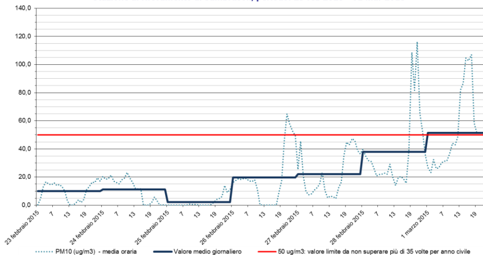
PM10 Stazione di rilevamento di Sambruson, periodo: 23 feb 2015 - 01 mar 2015
