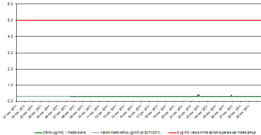
Benzene - C 6 H 6 Stazione di rilevamento ETL01322 in loc. Palù. periodo: 1 nov 2011-30 nov 2011
