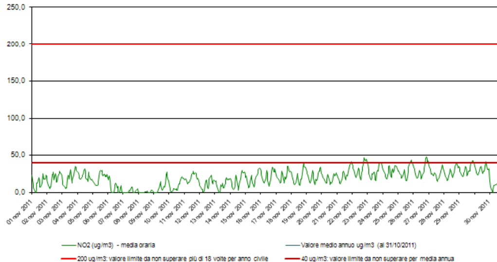
Biossido di azoto - NO 2 Stazione di rilevamento ETL01322 in loc. Palù, periodo: 1 nov 2011-30 nov 2011
