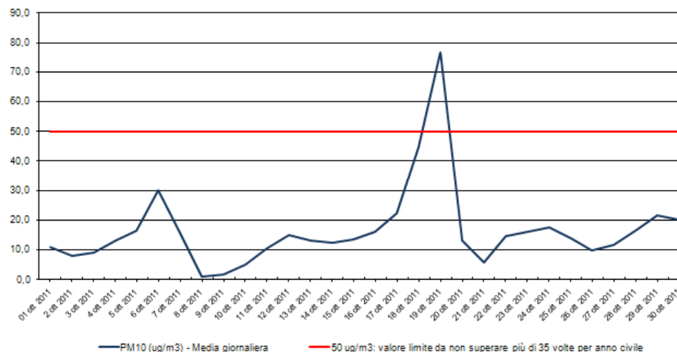
Stazione di rilevamento ETL01322 in loc. Palù, PM10 periodo: 1 ott 2011- 31 ott 2011
