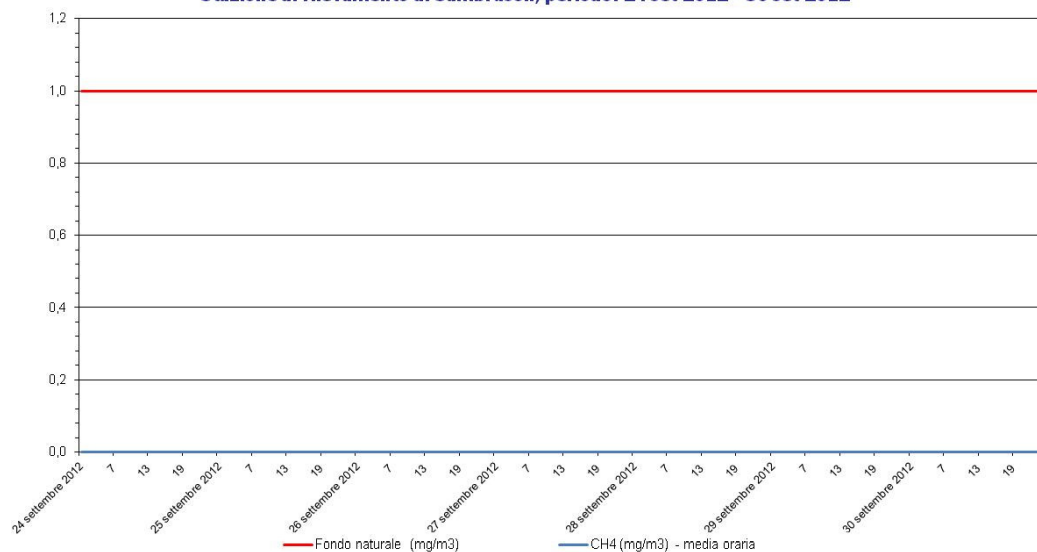
Metano - CH 4 Stazione di rilevamento di Sambruson, periodo: 24 set 2012 - 30 set 2012
