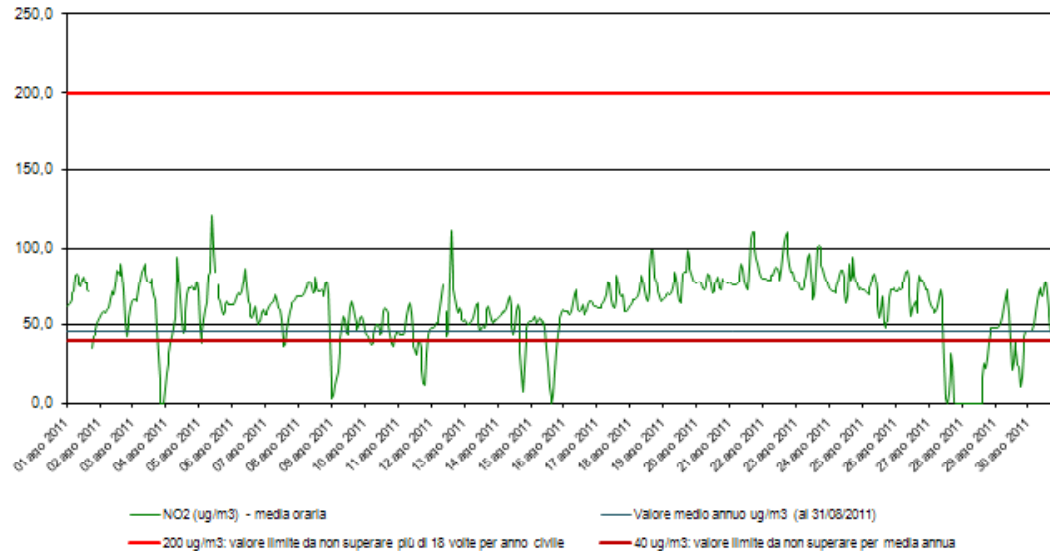
Biossido di azoto - NO 2 Stazione di rilevamento ETL01322 in loc. Palù, periodo: 1 ago 2011-31 ago 2011
