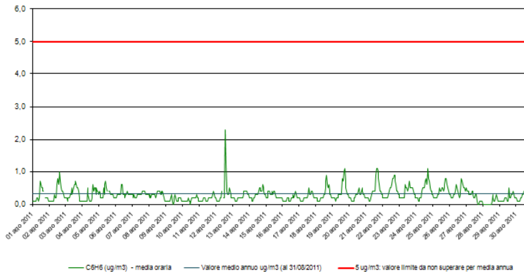
Benzene - C 6 H 6 Stazione di rilevamento ETL01322 in loc. Palù, periodo: 1 ago 2011-31 ago 2011
