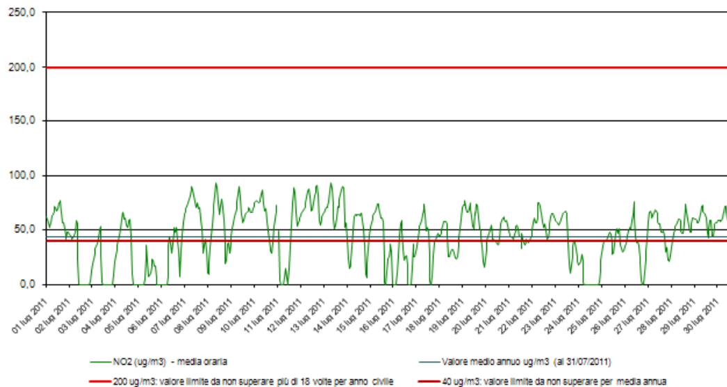
Biossido di azoto - NO 2 Stazione di rilevamento ETL01322 in loc. Palù, periodo: 1 lug 2011-31 lug 2011
