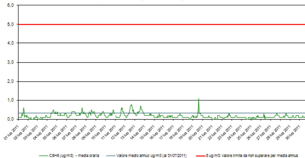
Benzene - C 6 H 6 Stazione di rilevamento ETL01322 in loc. Palù, periodo: 1 lug 2011-31 lug 2011
