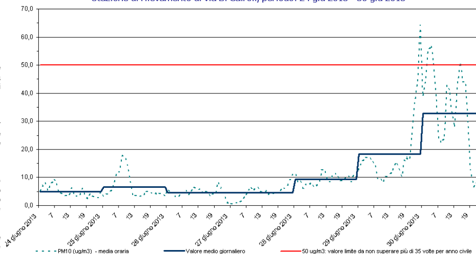
PM10 Stazione di rilevamento di via B. Cairoli, periodo: 24 giu 2013 - 30 giu 2013
