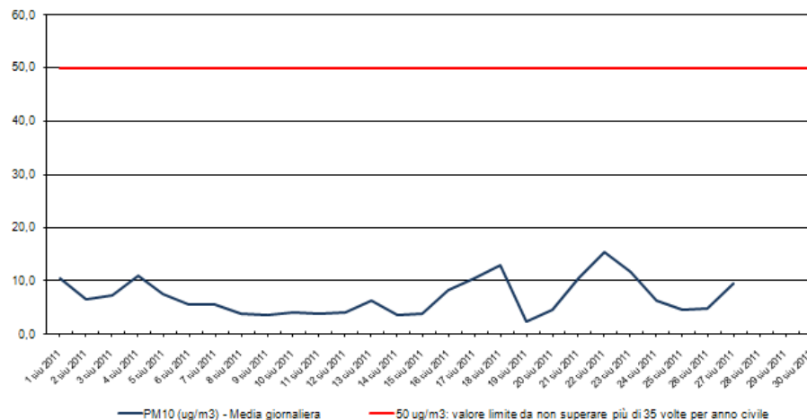
Stazione di rilevamento ETL01322 in loc. Palù, PM10 periodo: 1 giu 2011- 30 giu 2011
