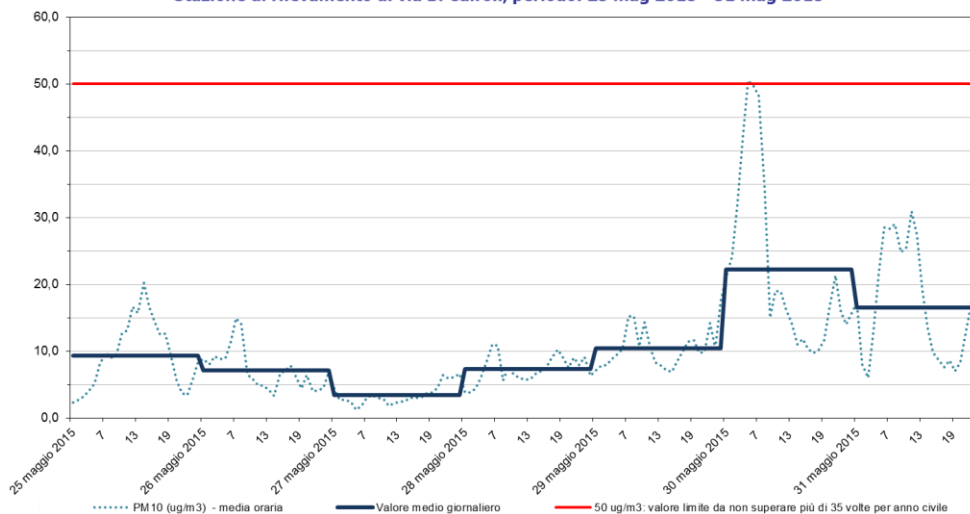
PM10 Stazione di rilevamento di via B. Cairoli, periodo: 25 mag 2015 - 31 mag 2015
