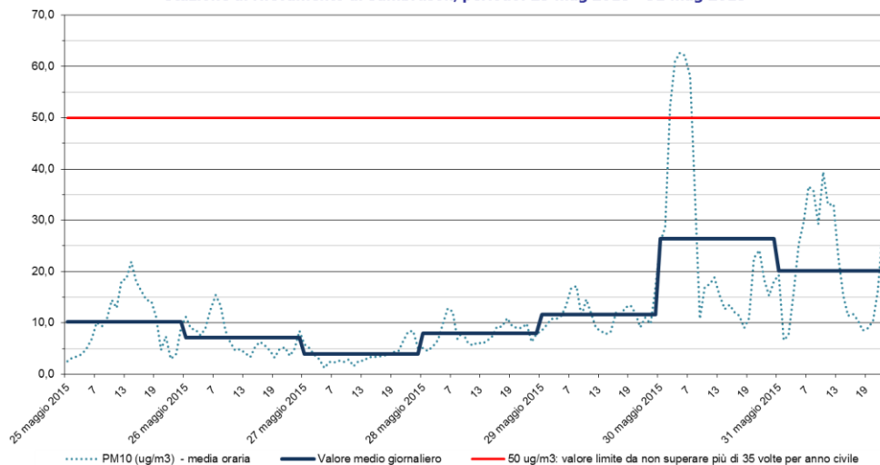
PM10 Stazione di rilevamento di Sambruson, periodo: 25 mag 2015 - 31 mag 2015
