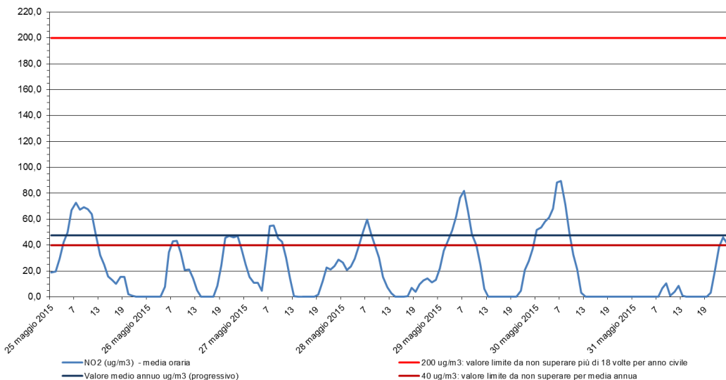
Biossido di azoto - NO 2 Stazione di rilevamento di via B. Cairoli, periodo: 25 mag 2015 - 31 mag 2015
