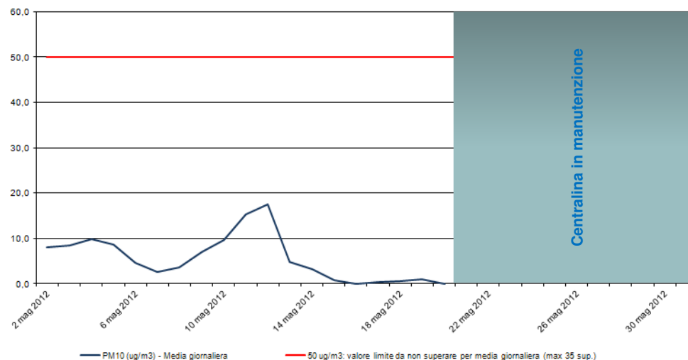
PM 10 Stazione di rilevamento ETL01322 in loc. Palù, periodo: 01 mag 2012- 31 mag 2012
