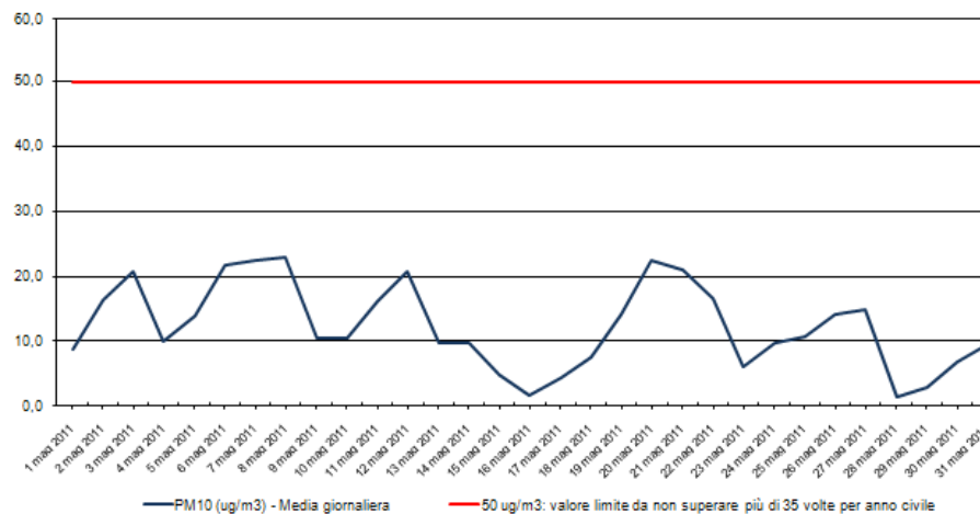
Stazione di rilevamento ETL01322 in loc. Palù, PM10 periodo: 1 mag 2011- 31 mag 2011
