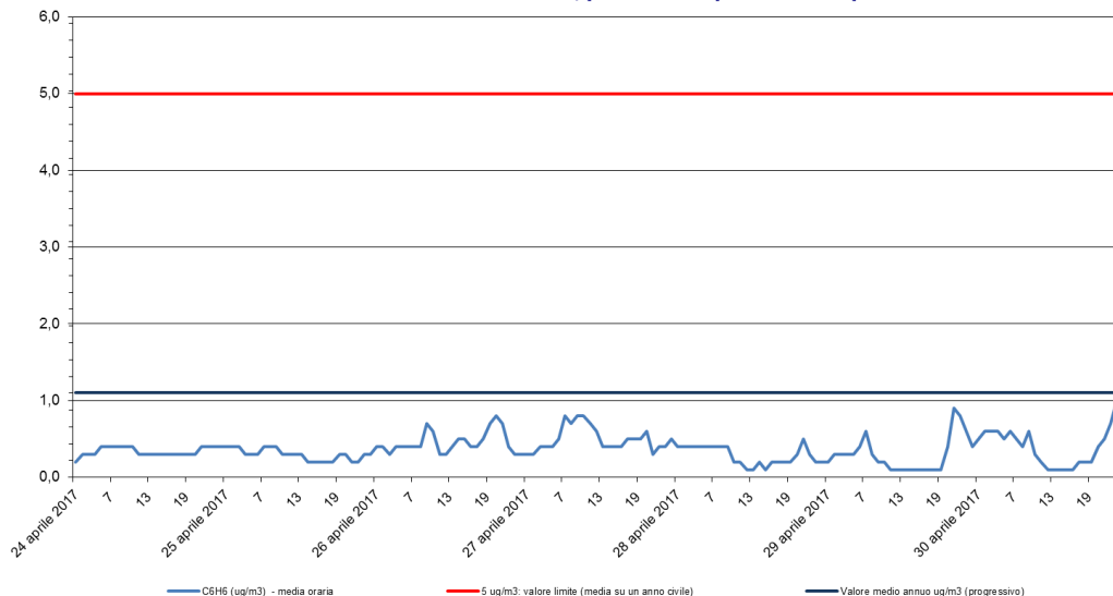
Benzene - C 6 H 6 Stazione di rilevamento di via B. Cairoli, periodo: 24 apr 2017 - 30 apr 2017
