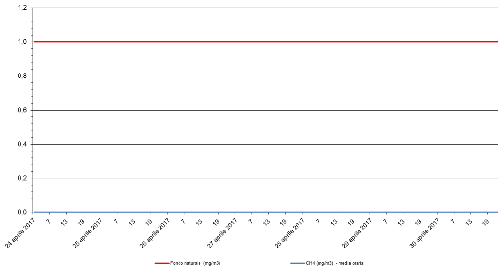
Metano - CH 4 Stazione di rilevamento di via B. Cairoli, periodo: 24 apr 2017 - 30 apr 2017
