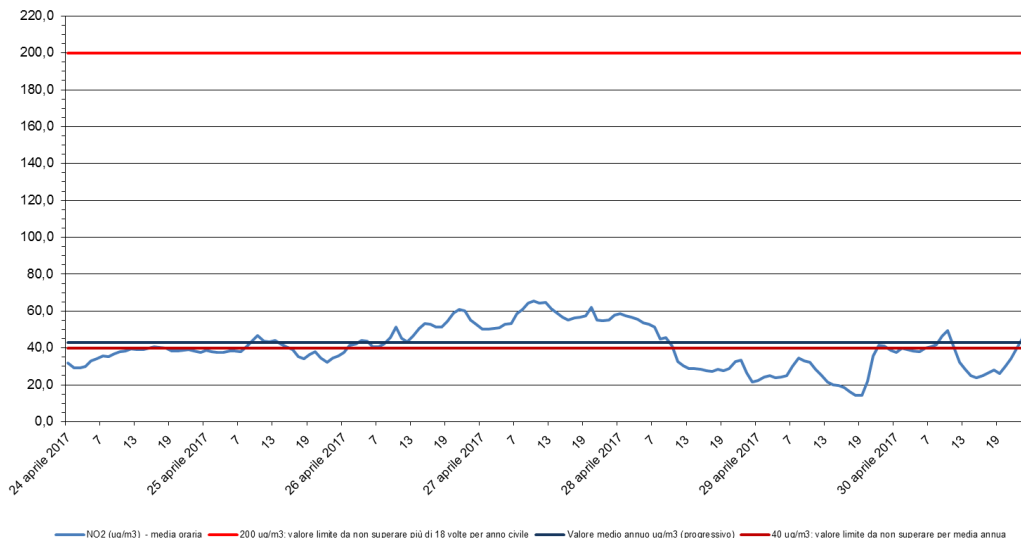
Biossido di azoto - NO 2 Stazione di rilevamento di via B. Cairoli, periodo: 24 apr 2017 - 30 apr 2017
