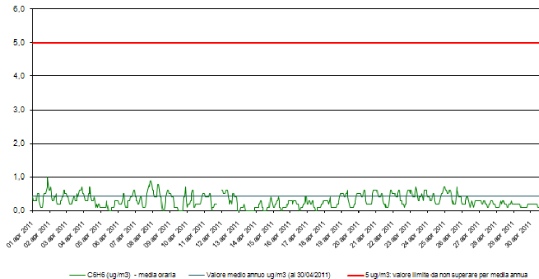
Benzene - C 6 H 6 Stazione di rilevamento ET101322 in loc. Paiù, periodo: 1 apr 2011-30 apr 2011
