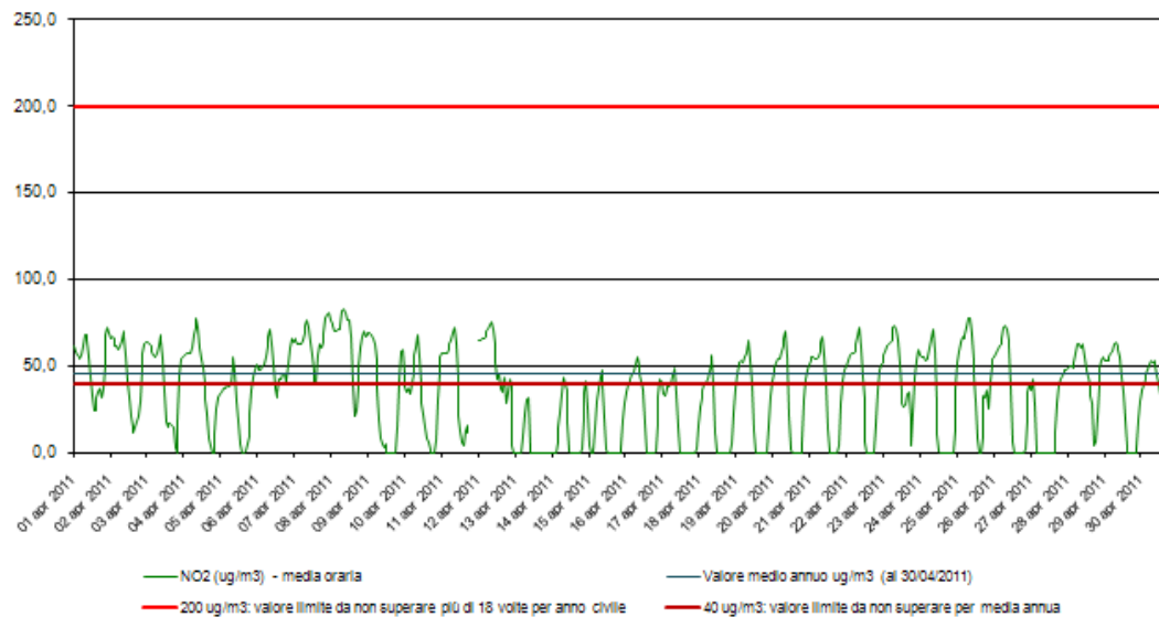
Biossido di azoto - NO 2 Stazione di rilevamento ETL01322 in loc. Palù, periodo: 1 apr 2011-30 apr 2011
