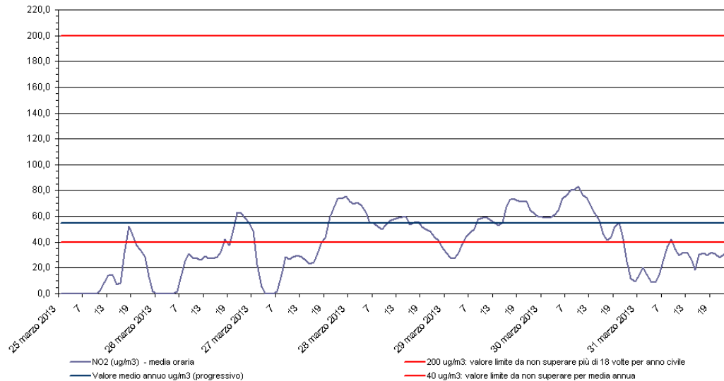
Biossido di azoto - NO 2 Stazione di rilevamento di via B. Cairoli, periodo: 25 mar 2013 - 31 mar 2013
