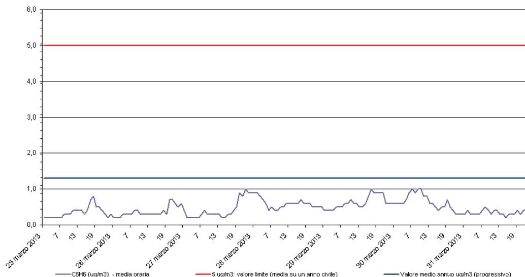
Benzene - C 6 H 6 Stazione di rilevamento di via B. Cairoli, periodo: 25 mar 2013 - 31 mar 2013
