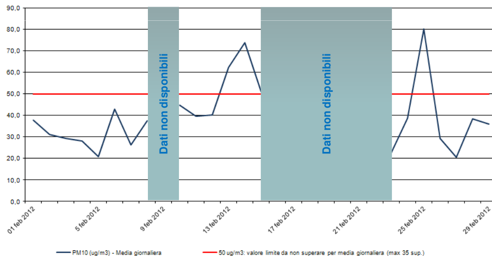
PM 10 Stazione di rilevamento ETL01322 in loc. Palù, periodo: 01 feb 2012- 29 feb 2012
