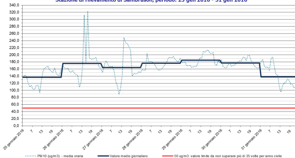
PM10 Stazione di rilevamento di Sambruson, periodo: 25 gen 2016 - 31 gen 2016
