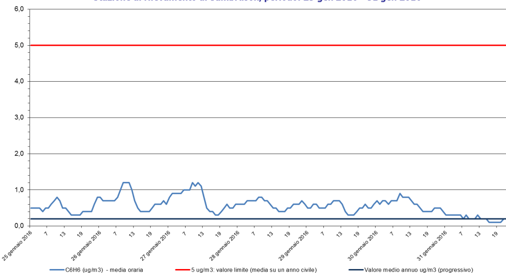
Benzene - C 6 H 6 Stazione di rilevamento di Sambruson, periodo: 25 gen 2016 - 31 gen 2016
