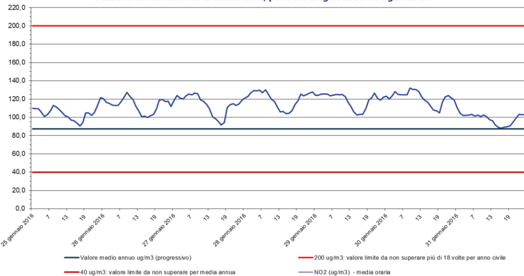
Biossido di azoto - NO 2 Stazione di rilevamento di Sambruson, periodo: 25 gen 2016 - 31 gen 2016
