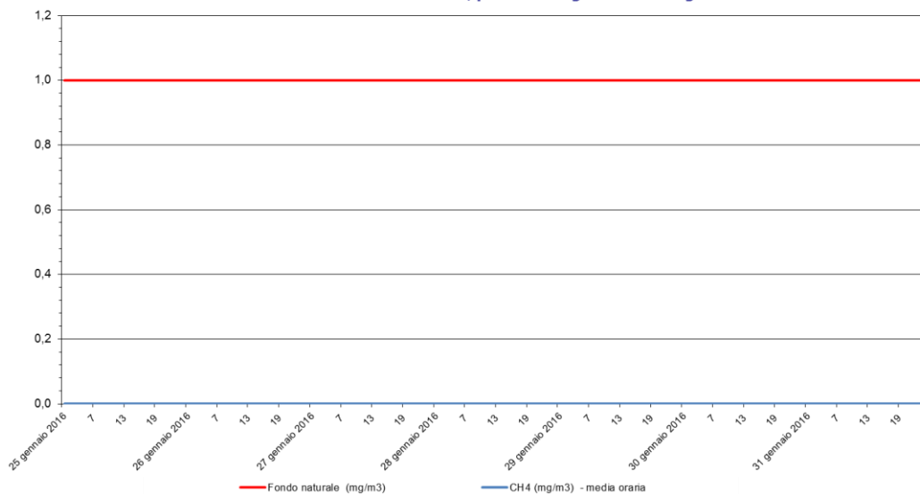
Metano - CH 4 Stazione di rilevamento di Sambruson, periodo: 25 gen 2016 - 31 gen 2016
