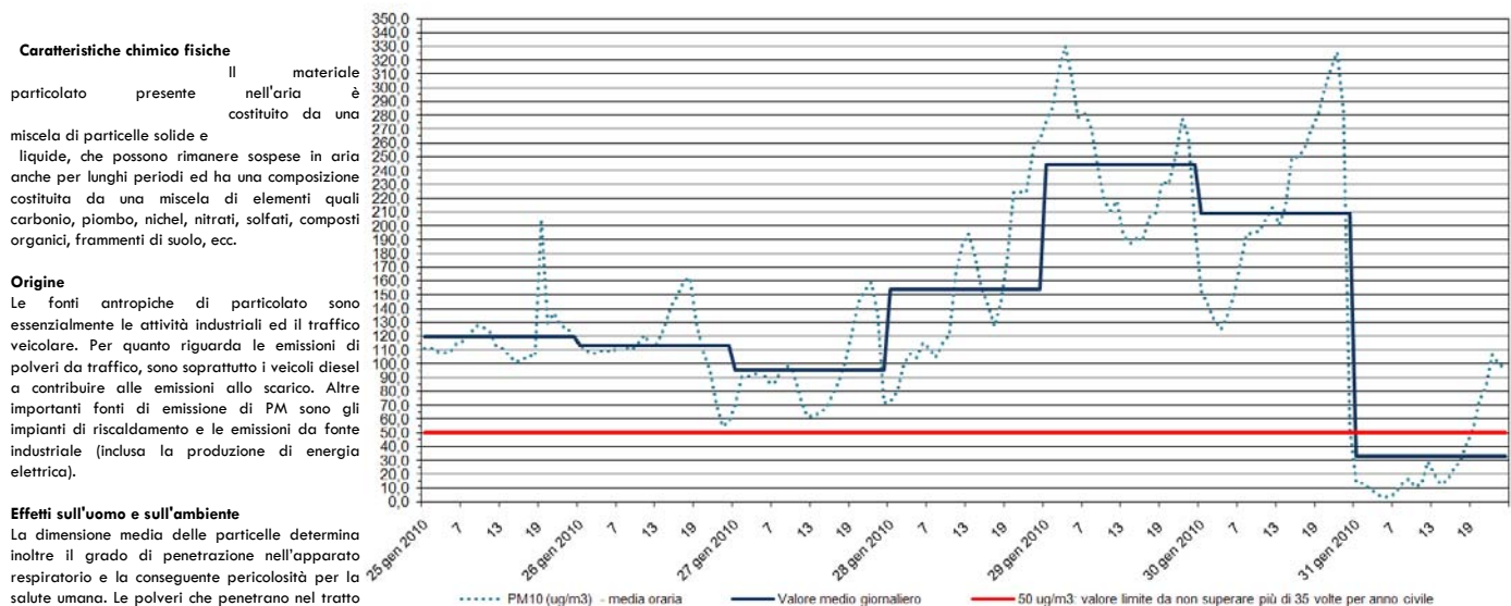
PM10 Stazione di rilevamento di via B. Cairoli, periodo: 25 gen 2010 - 31 gen 2010
