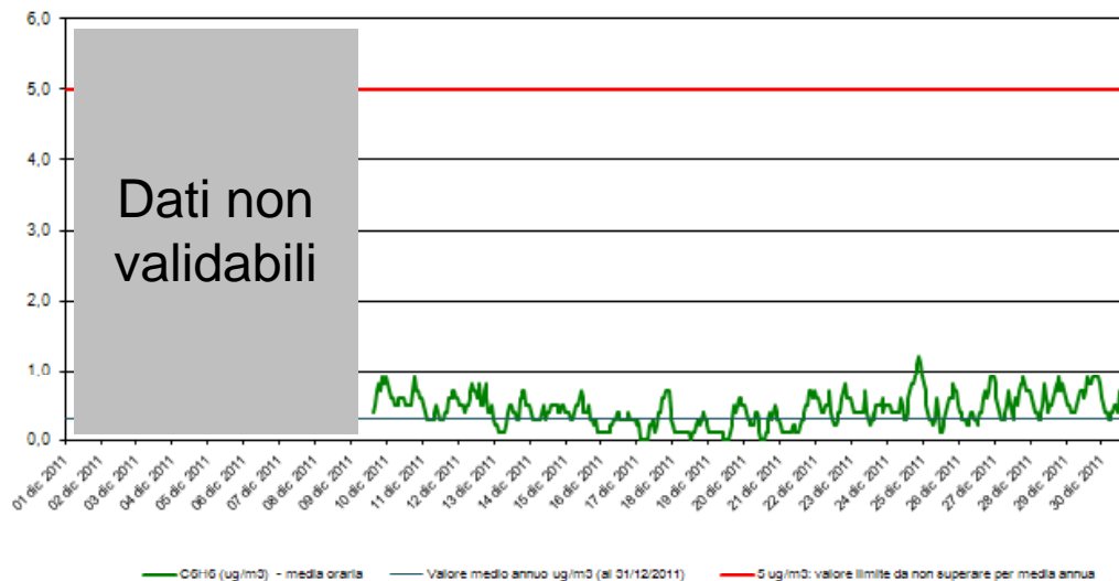
Benzene - C 6 H 6 Stazione di rilevamento ETL01322 in loc. Palù, periodo: 1 dic 2011-31 dic 2011
