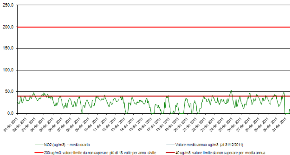
Biossido di azoto - NO2 Stazione di rilevamento ET101322 in loc. Palù, periodo: 1 dic 2011-31 dic 2011
