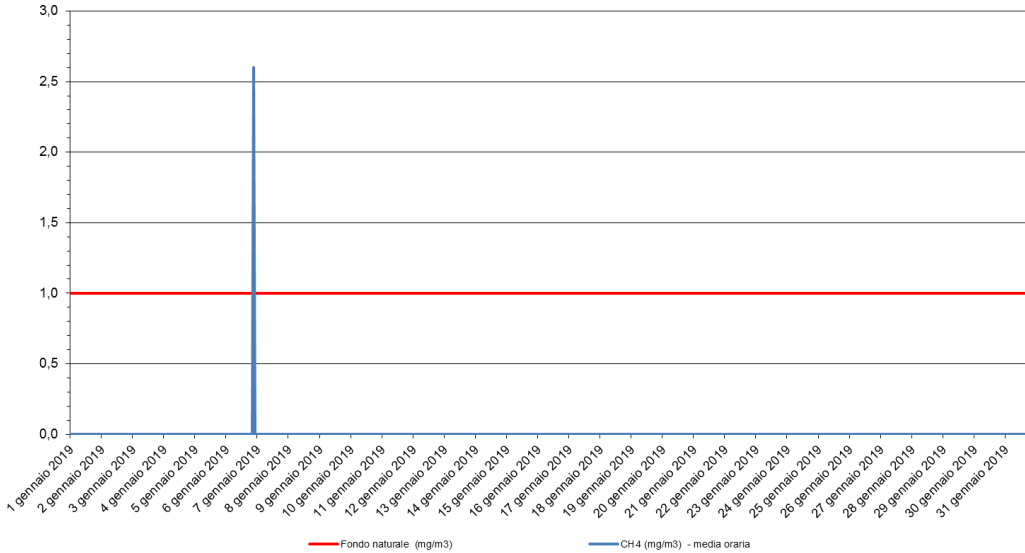
Metano - CH 4 Stazione di rilevamento di Sommacampagna, loc. Accademia - gennaio 2019
