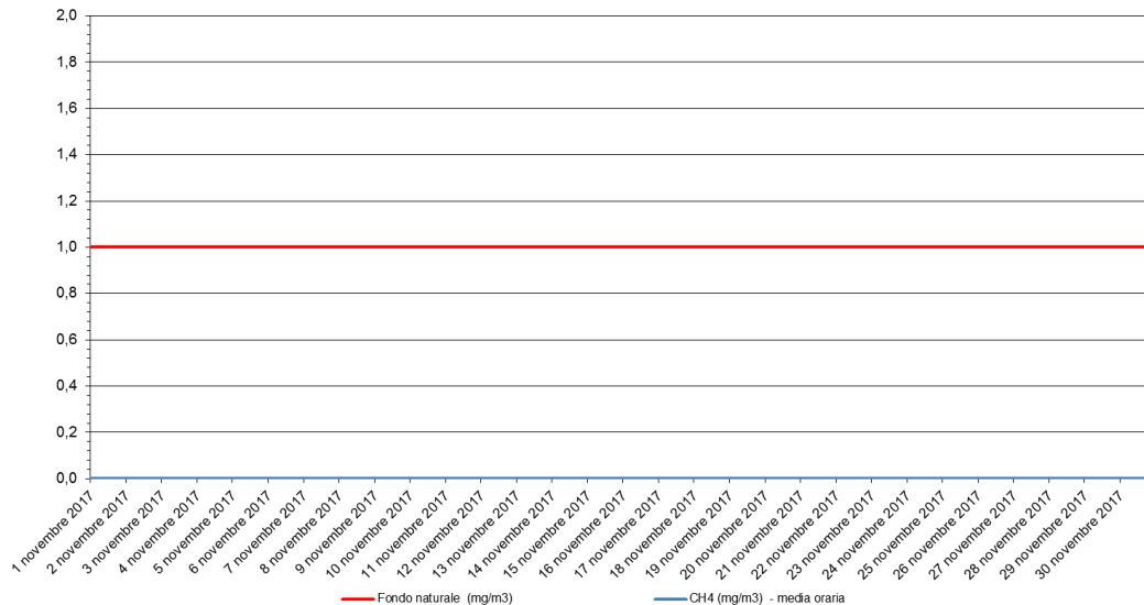
Metano - CH 4 Stazione di rilevamento di Sommacampagna, loc. Pirlar - novembre 2017
