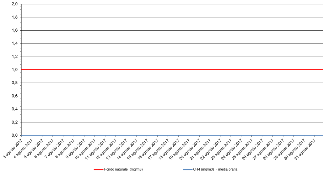
Metano - CH 4 Stazione di rilevamento di Sommacampagna, via Rezzola - agosto 2017
