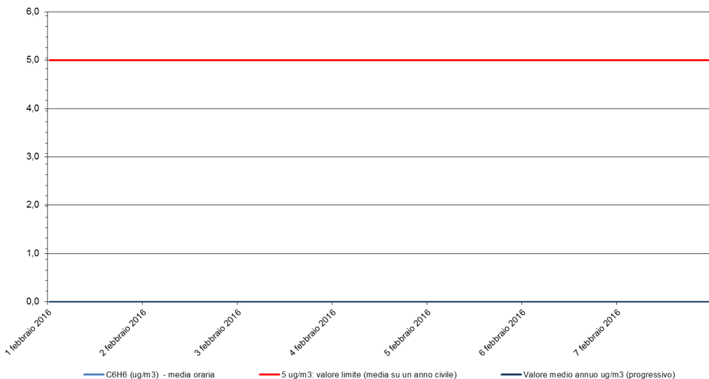
Benzene - C 6 H 6 Stazione di rilevamento di Custoza, strada Nuova - febbraio 2016
