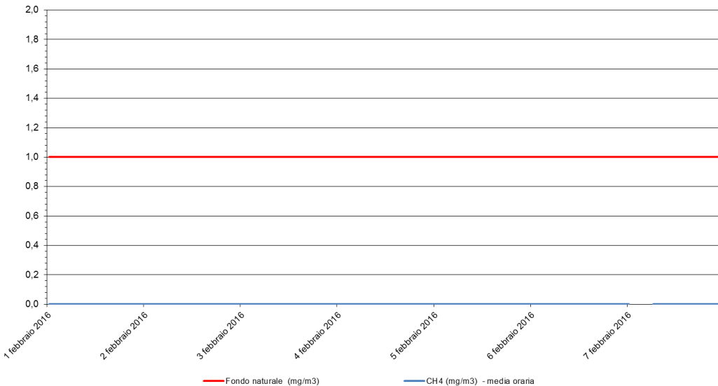
Metano - CH 4 Stazione di rilevamento di Custoza, strada Nuova - febbraio 2016
