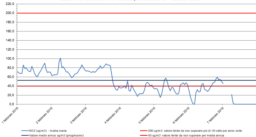
Biossido di azoto - NO 2 Stazione di rilevamento di Custoza, strada Nuova - febbraio 2016
